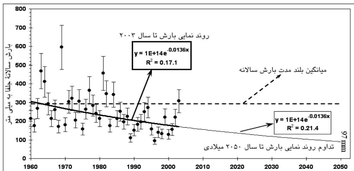
شکل ۷- پیش بینی روند نمایی بارش تا سال ۲۰۵۰ میلادی
