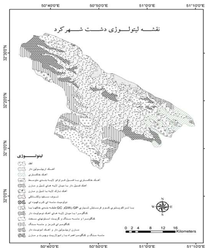
شکل ۳- نقشه لیتولوژی دشت شهرکرد
