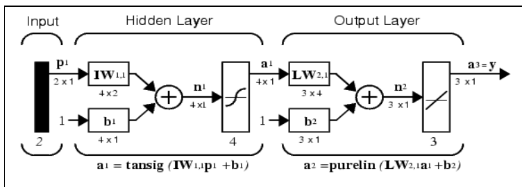
شکل شماره‌ی ۳: ساختار پرسپترون چندلایه با نرون‌های پنهان تانسیگ و نرون‌های خروجی با تابع خطی
