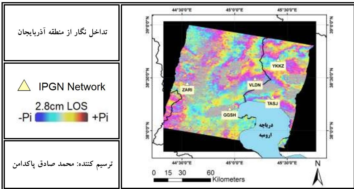
شکل ۵- تداخل نگار در منطقه آذربایجان Master: 2007-07-23 Slave: 2008-07-07
