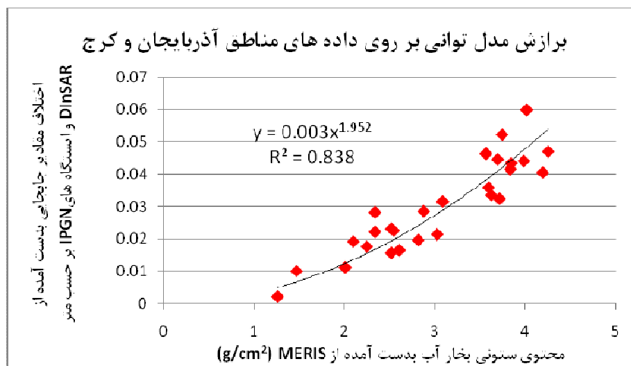
شکل ۷- برازش رگرسیون توانی بین مقادیر بخار آب MERIS و اختلاف مقادیر IPGN و DInSAR (آذربایجان و کرج)
