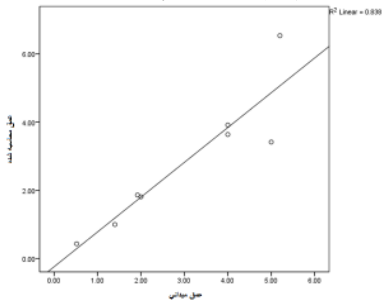
شکل (۳): نمودار ضریب همبستگی بین عمق میدانی و عمق محاسبه شده (منبع: نگارندگان)
