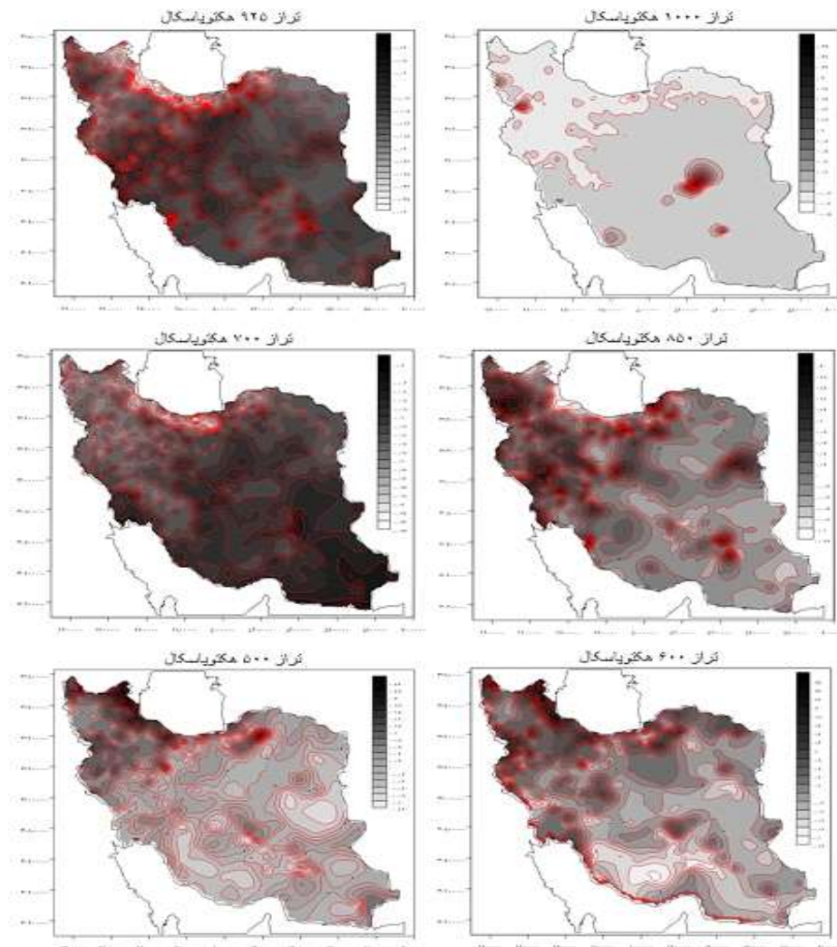
شکل (۵) نقشه همبستگی تعداد چرخندها با بارش یاخته‌ای کشور در ترازهای مختلف
