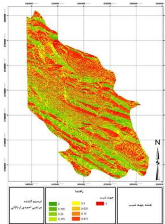
شکل (۸) نقشه جهت شیب
