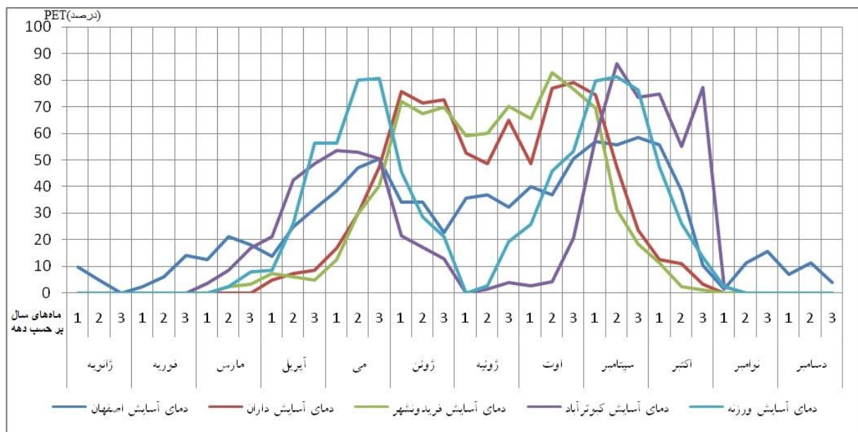
شکل 6. نمودار مقایسه روزانه درصد آسایش اقلیمی ( 18 < PET^{\circ}C < 29 ) ایستگاه‌های مطالعه‌شده
