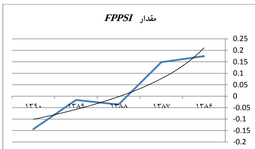
شکل ۹. میزان FPPSI آلودگی شهر اصفهان در سال‌های ۱۳۸۶-۱۳۹۰
