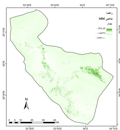
شکل ۲۰. نتایج NDVI برای بارزسازی پوشش گیاهی
