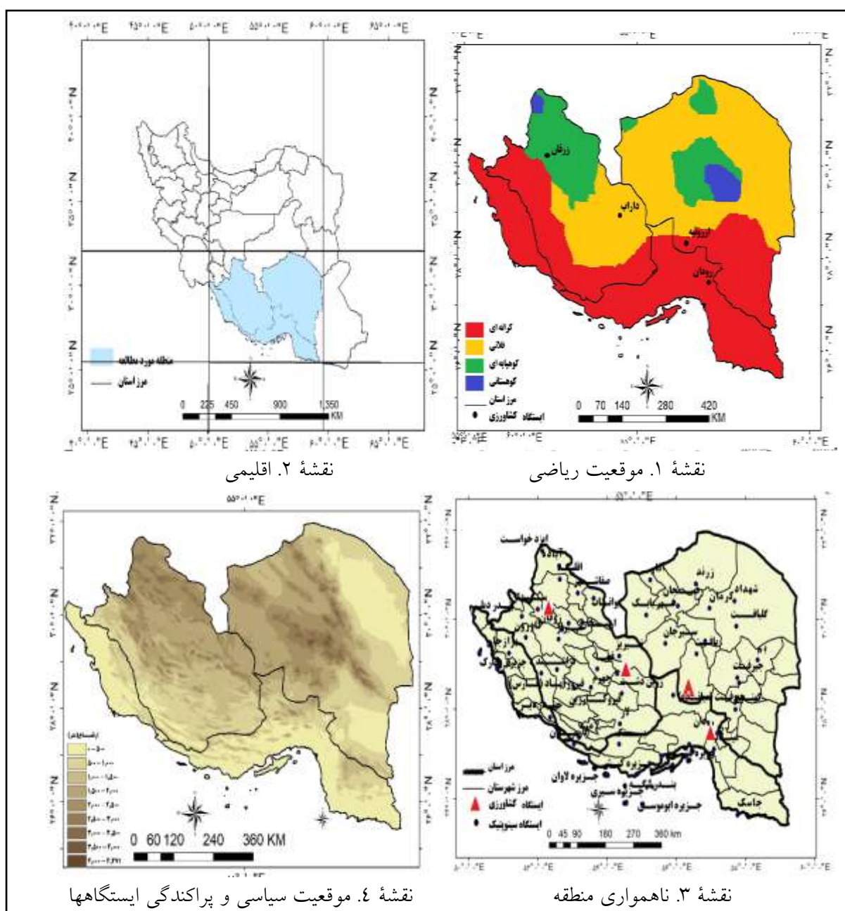
شکل ۱. نقشه‌های موقعیت ریاضی، اقلیمی (اقتباس از نقشه ناحیه‌بندی اقلیمی ایران، مسعودیان، ۱۳۹۰)، ناهماری، موقعیت سیاسی و پراکندگی ایستگاهها
