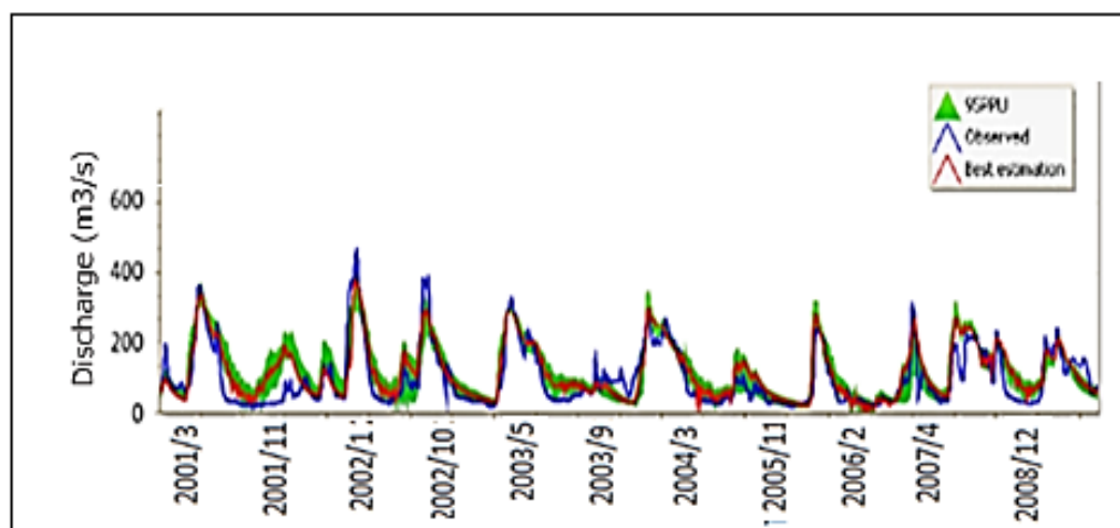
شکل (۹) منحنی رابطه بین مقادیر رواناب شبیه‌سازی شده و مشاهداتی دوره واسنجی (۲۰۰۱-۲۰۰۸) در حوضه آبریز قره‌چای (منبع: نویسندگان، ۱۴۰۱)
