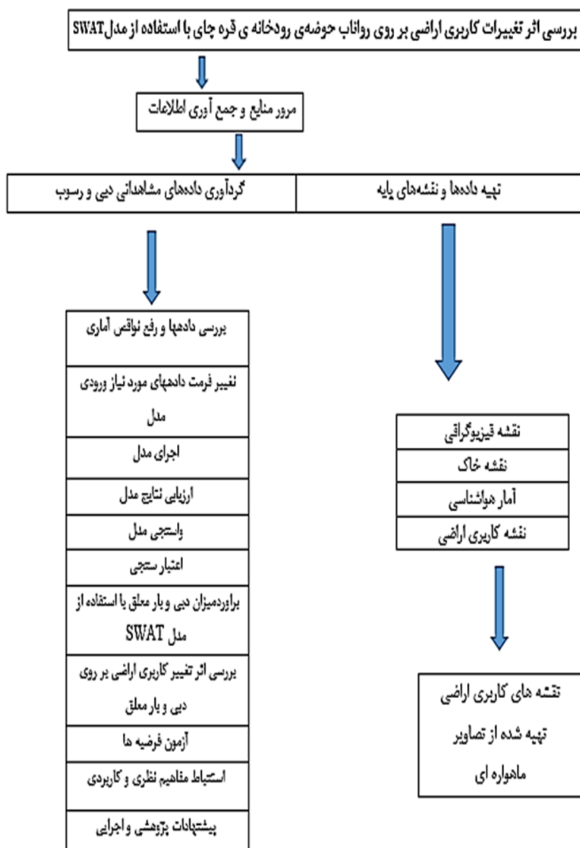
شکل (۳) نمودار جریان‌ی مراحل انجام مدل SWAT در پژوهش حاضر (منبع: نویسندگان، ۱۴۰۱)
