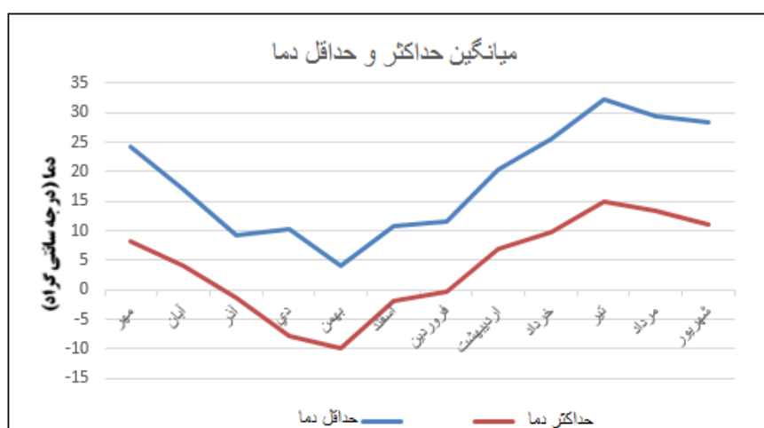
شکل (۱) میانگین بیشترین و کمترین دما، کمترین دمای مطلق، بیشترین دمای مطلق و میانگین بارش ماهانه ایستگاه یلفان (منبع: نویسندگان، ۱۴۰۱)
