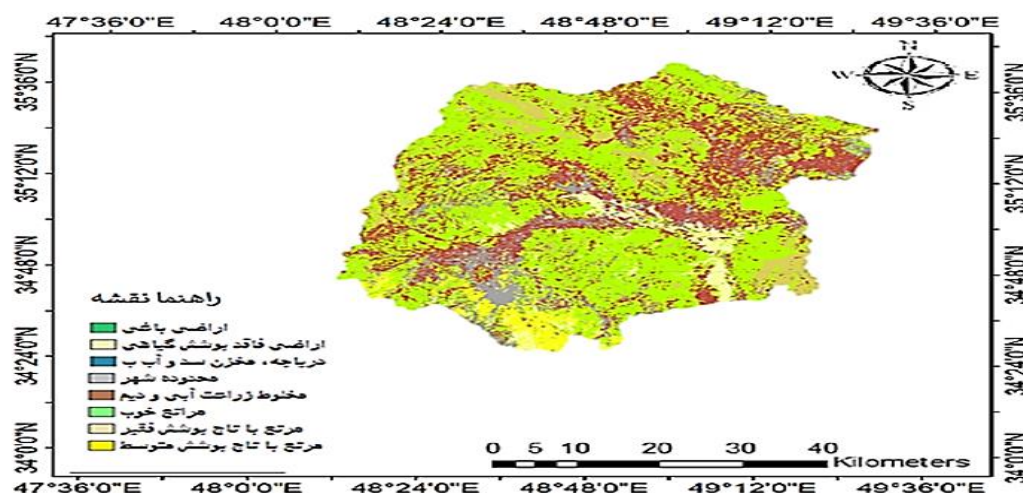
شکل (۷) تغییرات کاربری اراضی در حوضه آبریز قره‌چای در سال ۱۳۹۹ نسبت به سال ۱۳۸۰ (منبع: نویسندگان، ۱۴۰۱)
