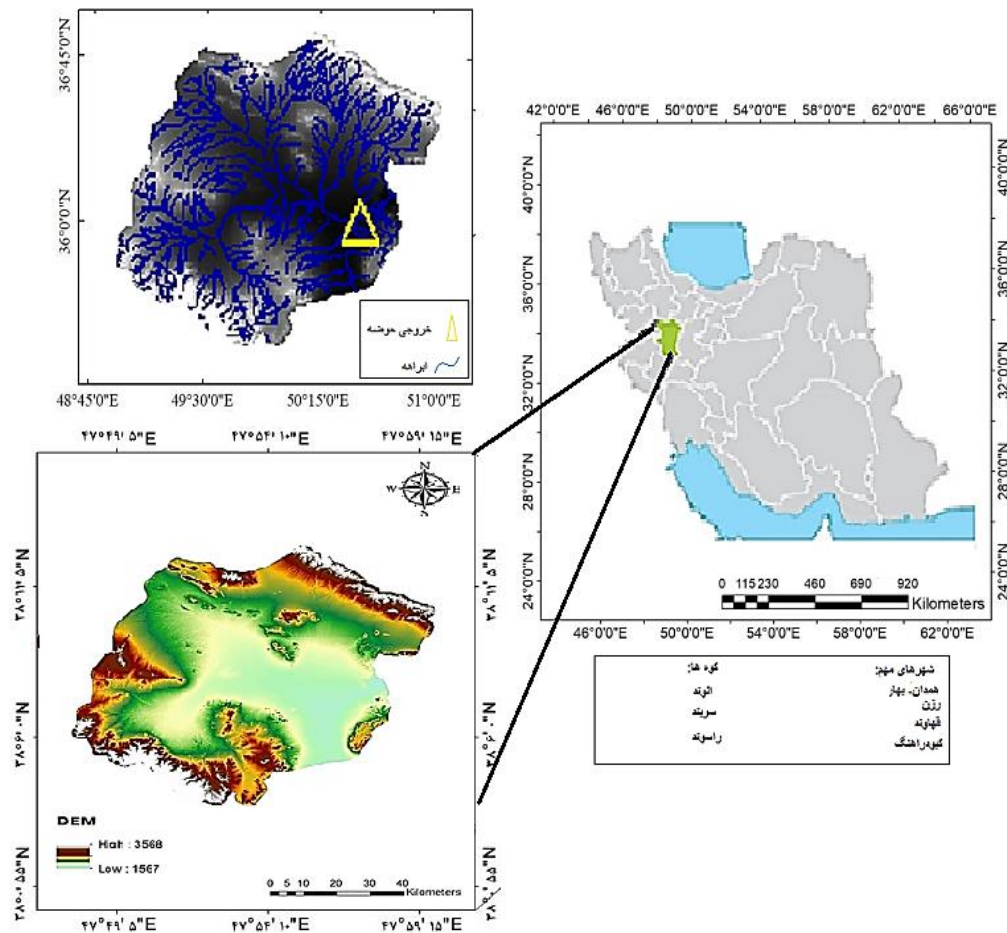
شکل (۲) موقعیت حوضه قره‌چای در استان همدان (منبع: نویسندگان، ۱۴۰۱)
