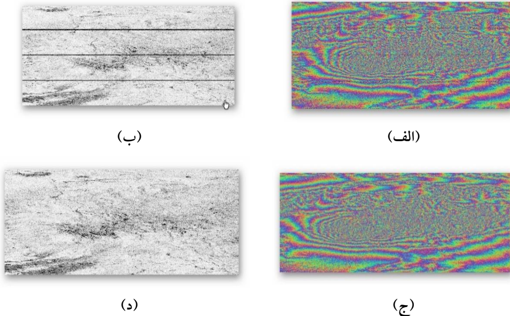
شکل (۳) (الف) تصویر فاز دارای نوار؛ (ب) تصویر کوهرنسی دارای نوار؛ (ج) تصویر فاز تصحیح نوارشده؛ (د) تصویر کوهرنسی نواری شده
