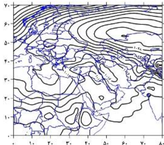
شکل ۸- الگوی گردشی چهارم فشار تراز دریا در روزهای گرد و غباری
