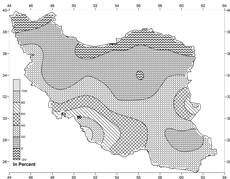
شکل (۳): شبیه سازی میانگین درصد تغییرات سالانه بارش نسبت به مانگن دراز مدت ۱۹۶۱ تا ۱۹۹۰، با استفاده از نتایج
