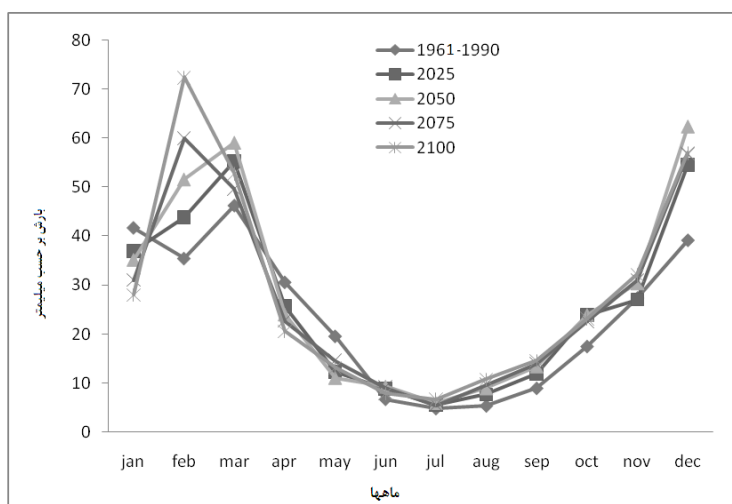
شکل (۵): تغییرات ماهانه مقادیر مشاهداتی و شبیه سازی شده بارش کشور در ادوار مختلف
