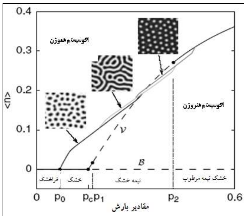
شکل ۷: ارتباط بیومس (n) و بارش (p): خط معرف B حالت یا وضعیت بایر است، جاییکه بیومس تقریباً برابر با صفر است (n=0). منحنی v مشخص کننده الگوی یکنواخت پوشش گیاهی است. به طور کلی الگوهای پوشش به عنوان یک شاخص تغییرات محیطی مشخص کننده وضعیت سیستم و شرایط اقلیمی است (اقتباس از ون هاردنبرگ و همکاران، ۲۰۰۱، با اندکی تغییر).
