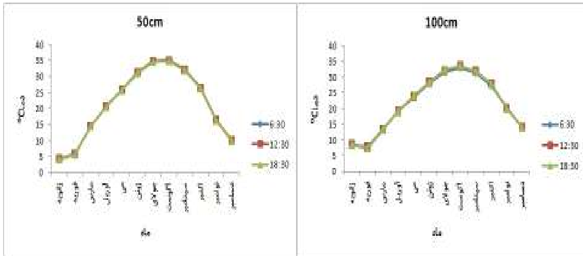
شکل ۲) الگوی رفتار ماهانه دمای اعماق مختلف خاک
