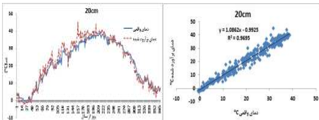
شکل ۵- الف) میانگین دمای روزانه برآورد شده و واقعی ب) همبستگی بین آنها در عمق ۲۰ سانتیمتری
