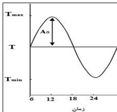
شکل (۱) نوسانات آرمانی دما در خاک
