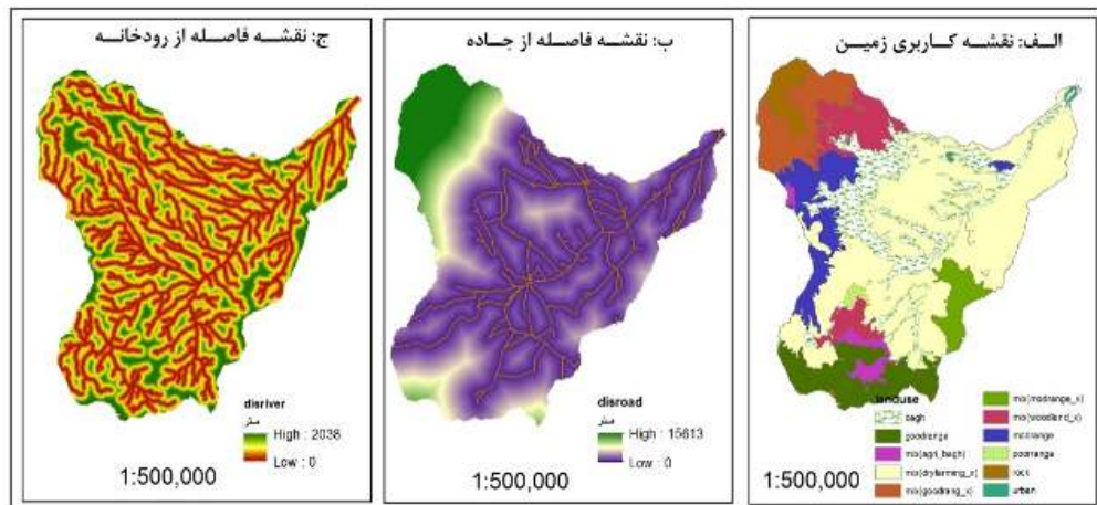
شکل ۷- نقشه لایه‌ها الف) کاربری زمین (منبع نگارندگان: استخراج از تصویر ماهواره‌ای). ب) فاصله از جاده. ج)
