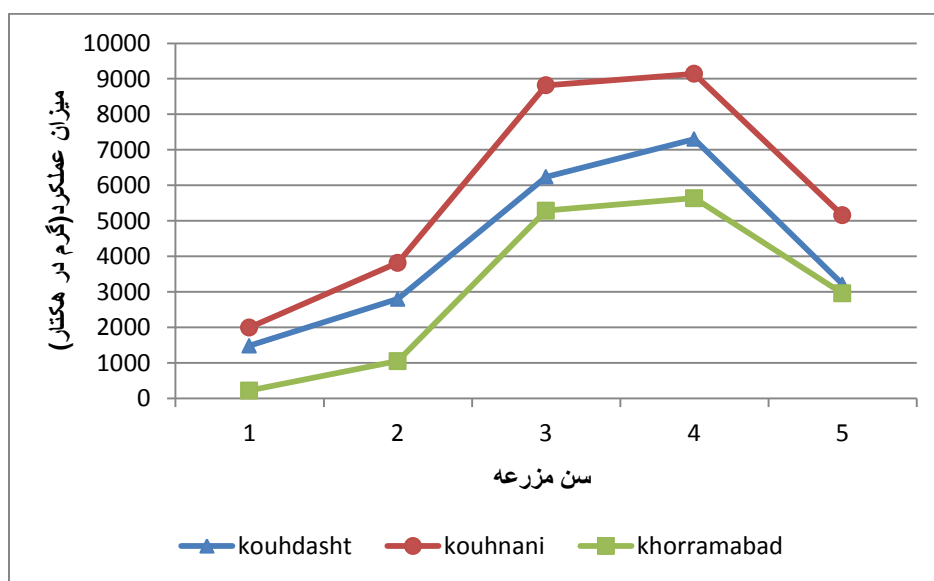
شکل ۶. نمودار عملکرد محصول گیاه زعفران در مناطق مطالعه‌شده در سال ۱۳۹۷
