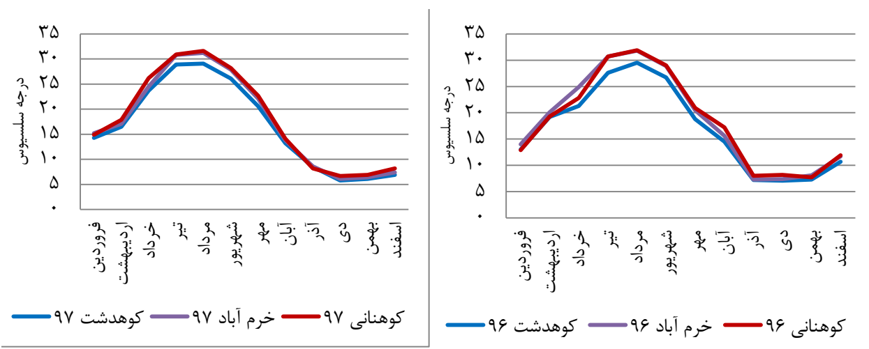
شکل ۲. نمودار میانگین دمای ماهانه ایستگاه‌های طی دو سال ۱۳۹۷ و ۱۳۹۶
