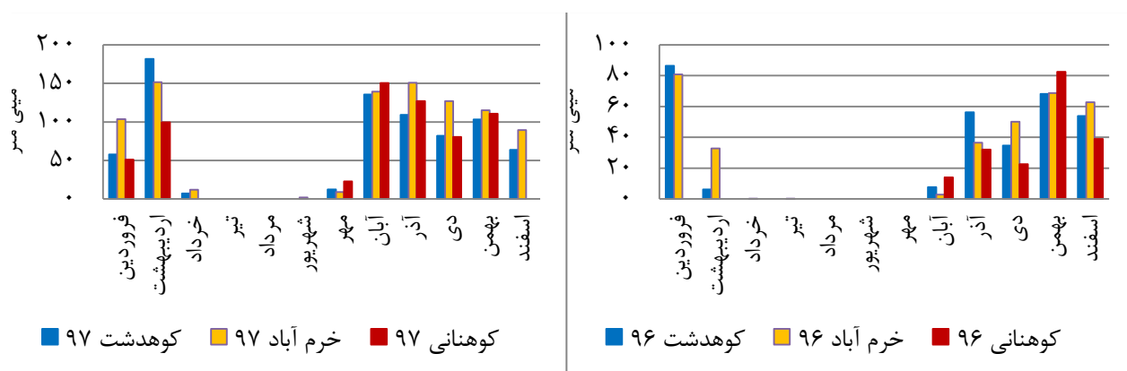
شکل ۳. نمودار میانگین بارش ماهانه ایستگاه‌ها در سال ۱۳۹۷ و ۱۳۹۶
