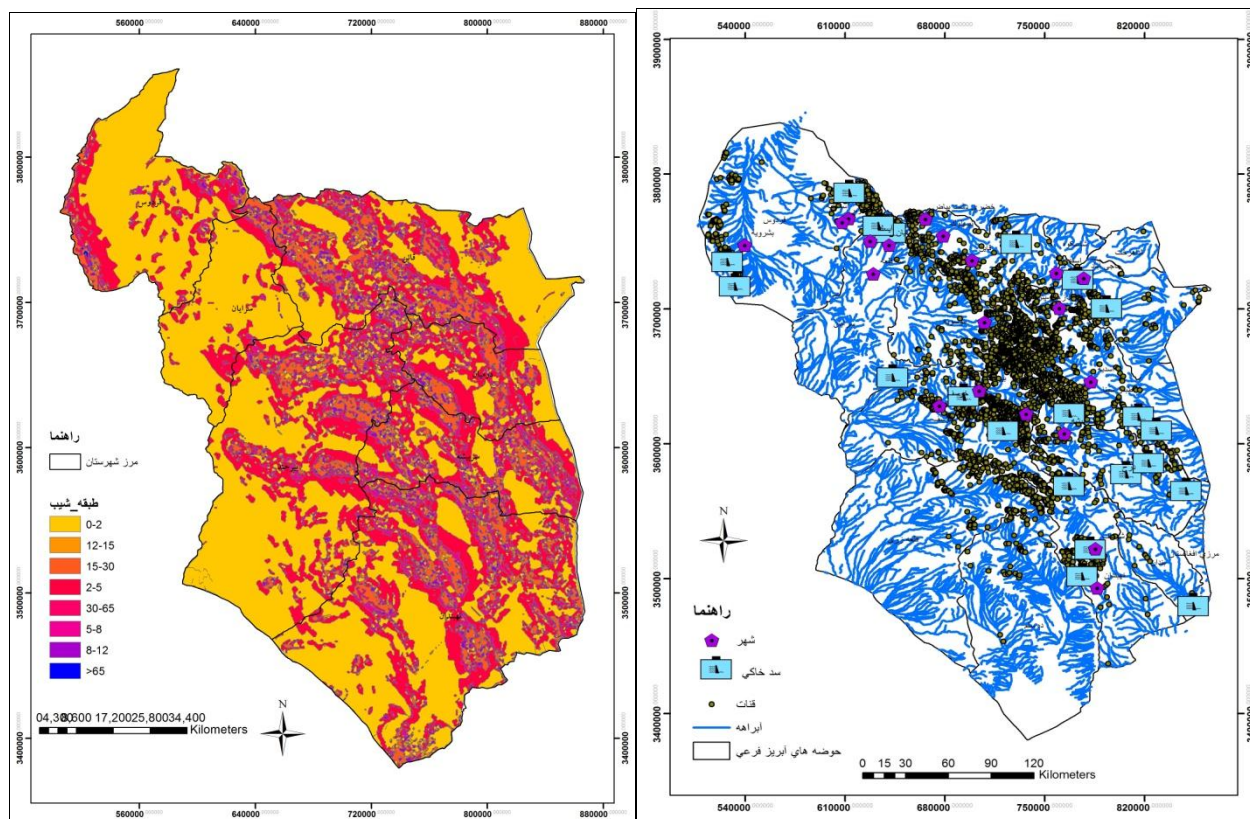
شکل ۶. نقشه طبقات شیب استان خراسان جنوبی
